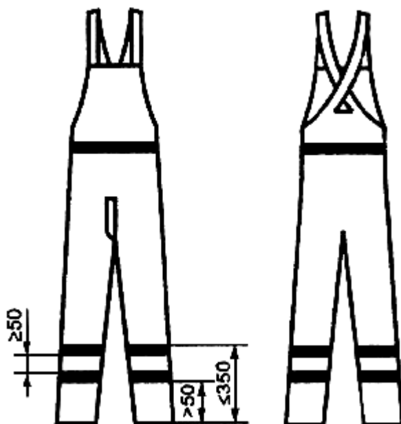
Рисунок Б.8 - Полукомбинезон
