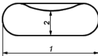
Рисунок 12 - Линейные измерения подследников
